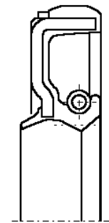
シール断面
